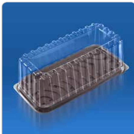
کد: ۵۰۲۲۲۸ ظرف کیک رولتی کامل تعداد در کارتن: ۷۵ عدد ابعاد: ۳۷۵*۱۸۳*۱۱۰
